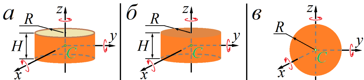
Рис. 8.11. Тела, для которых представлены формулы (8.33)– (8.35) центральных моментов инерции:
