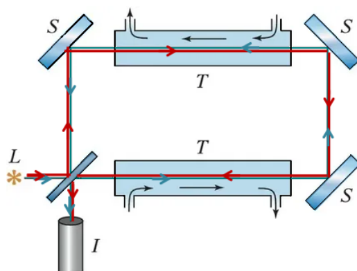
Рис. 9.2. Опыт Физо
