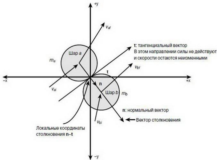
Рис. 7.12. Нецентральный удар
