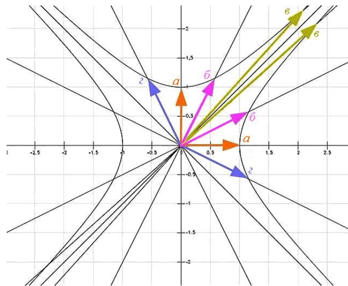
Рис. 9.13. Единичные векторы x и tv разных ИСО. a - \beta=0 ; b - \beta=0,5 ; c - \beta=0,9 ; z - \beta=-0,5
