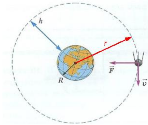
Рис. 7.11. Орбитальное движение
