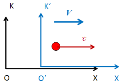
Рис. 9.10. Сложение скоростей
